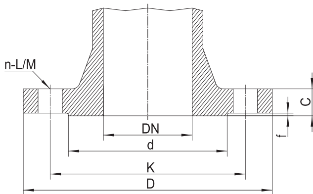
Рис. 18 Характеристики фланцев
