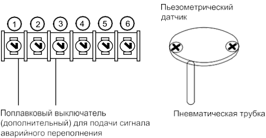
Рис. 13 Подключение реле уровня, порта диспетчеризации, внешней аварийной сигнализации
