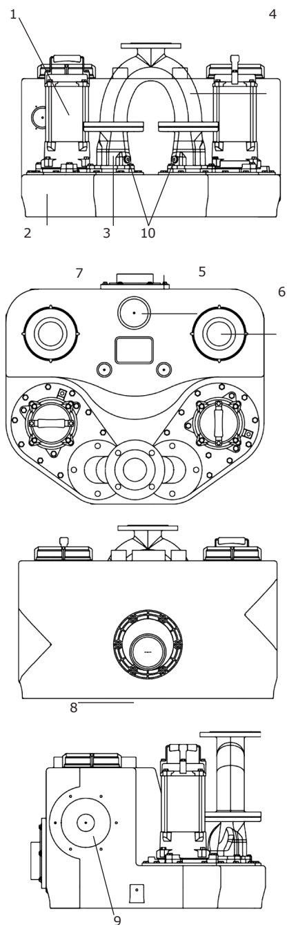
Рис. 1 Компоненты установки Prolift
