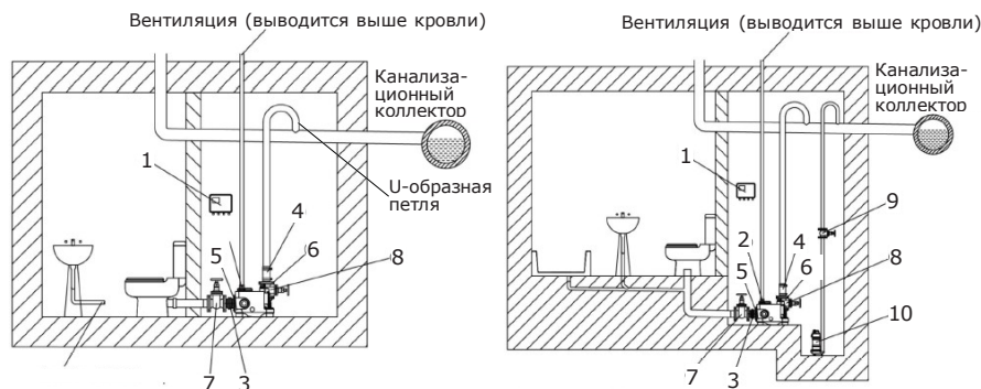
Рис. 2 Схема монтажа с прямым подключением (слева) и в приемке (справа)
