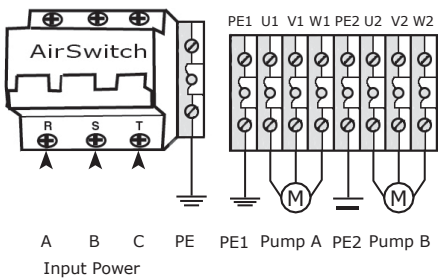
Рис. 12 Схема внешних подключений
