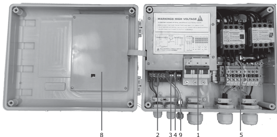
Рис. 11 Внешний вид шкафа управления
