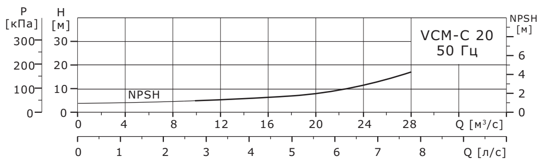
Рис. 23 Кривая NPSH для VCM-C 20
