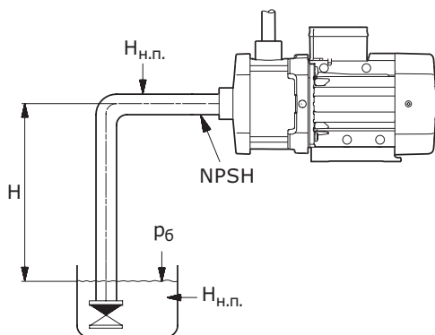
Рис. 10 Минимальное давление на входе
