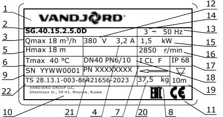
Рис. 2 Фирменная табличка
