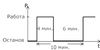
Рис. 7 Режим работы S3
