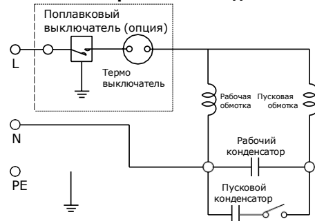
Рис. 3 Схема соединений для насосов с однофазными электродвигателями
