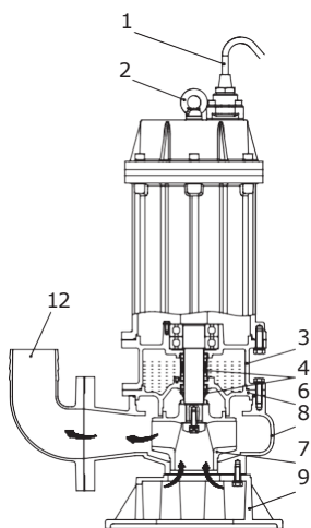
Рис. 3 VSL, 7,5 – 11,0 кВт, 2-полюсный
