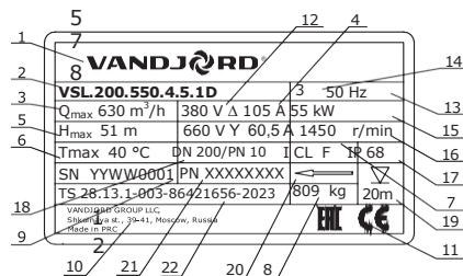
Рис. 9 Фирменная табличка
