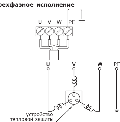
Рис. 13 Схема подключения 3-фазного насоса, прямой пуск, схема соединения обмотки «звезда». Электродвигатель со встроенным термодатчиком
