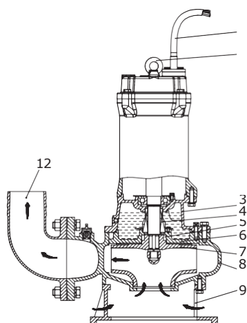
Рис. 4 VSL, 2,2 – 3,7 кВт, 4-полюсный
