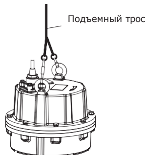
Рис. 10 Точки подъема (насос 1,5...90 кВт)
