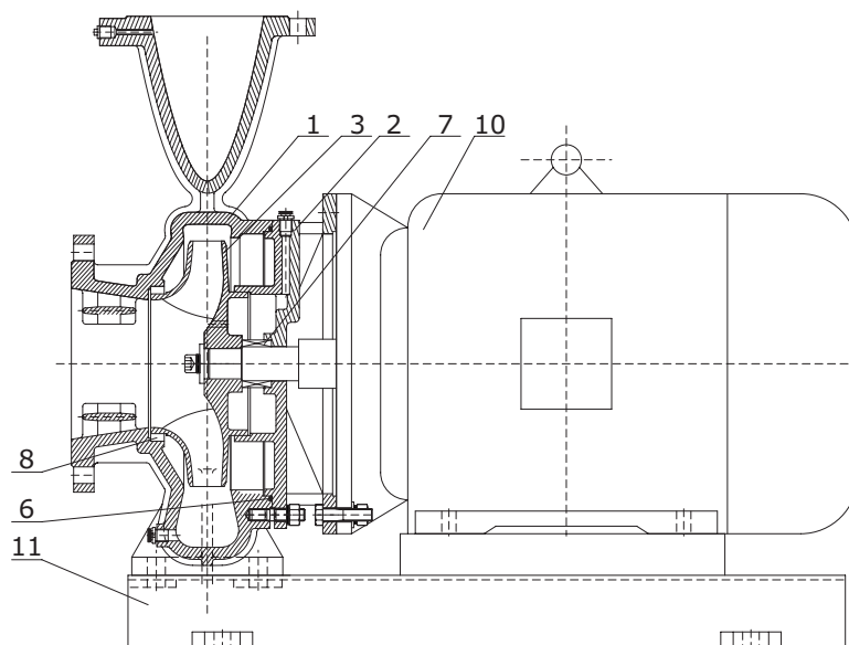
Рис. 1 Насос NBV в разрезе (конструкция с удлиненным валом двигателя)
