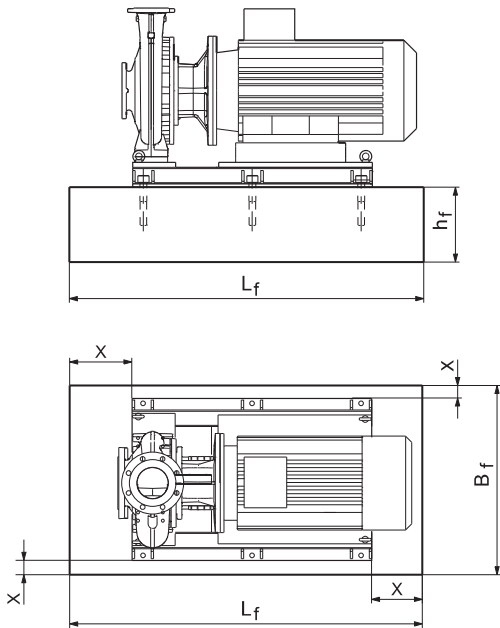
Рис. 10 Фундамент, X = мин. 100 мм
