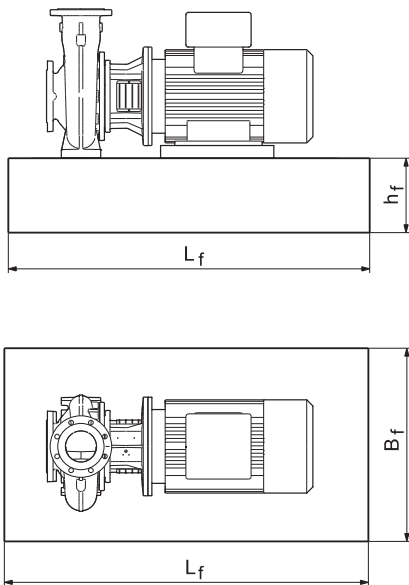
Рис. 9 Фундамент
