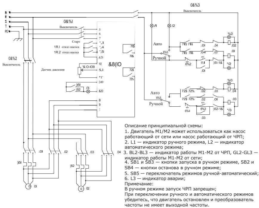
Рис. 25 Принципиальная схема 11-400 кВт
