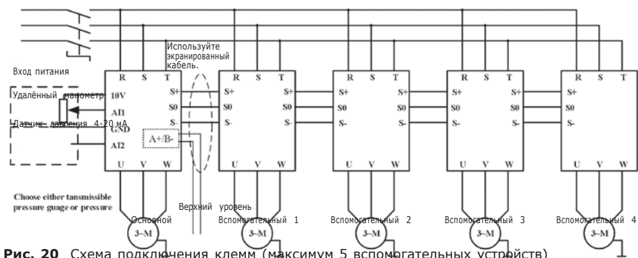
Рис. 20 Схема подключения клемм (максимум 5 вспомогательных устройств)
