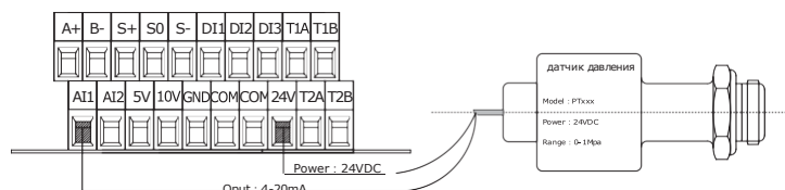
Рис. 17 0,75–7,5 кВт схема подключения двухпроводного датчика давления
