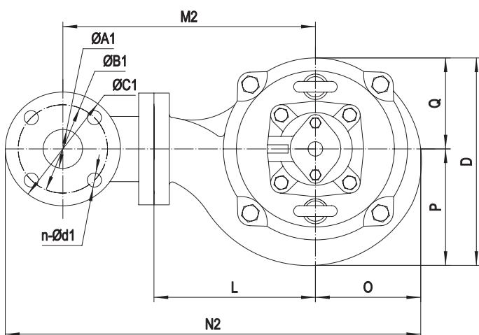
Размеры напорного патрубка насоса
